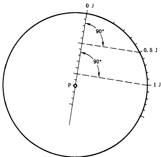
图 B.6 分度盘“f”
